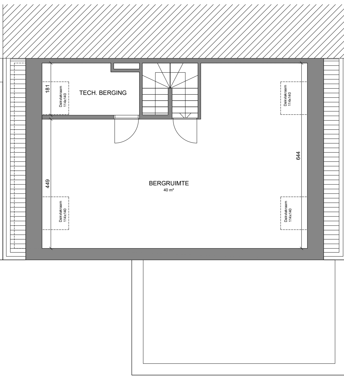
DAHLIASTRAAT 18 (U43) - zolder
